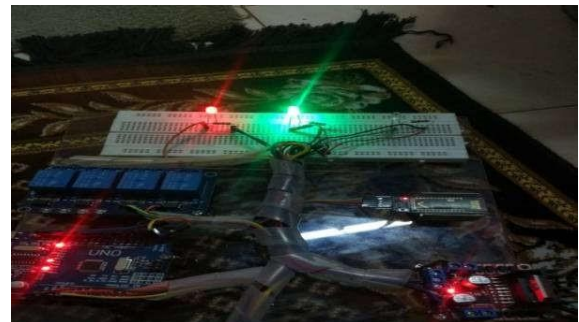
Gambar 7. Rangkaian Pengujian Otomatis Spray Desinfektan Kandang Ayam Dengan Android Berbasis Arduino Uno
