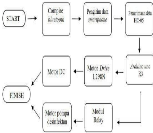
Gambar 1. Blok Diagram Pengembangan Sistem
